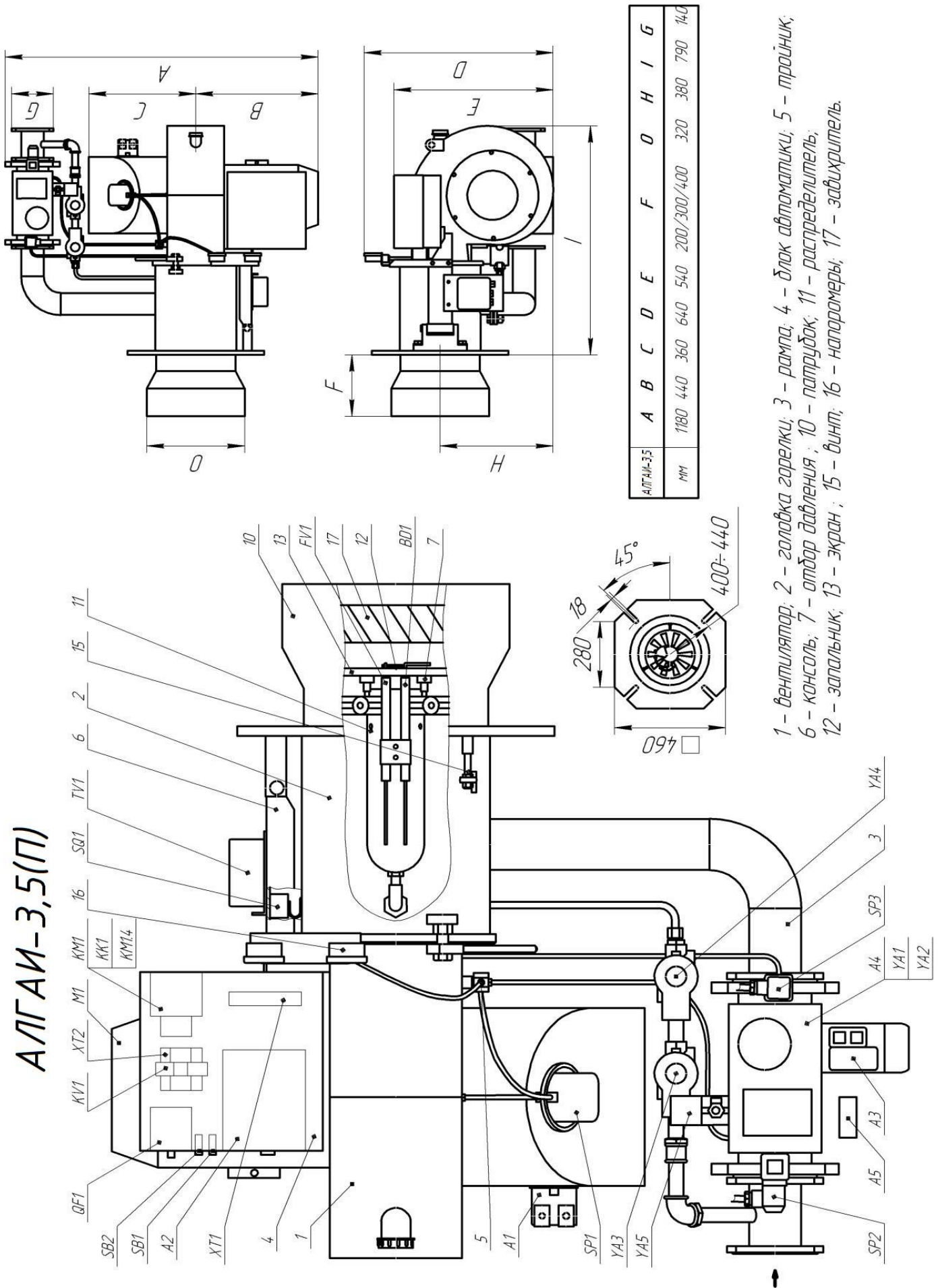
Рисунок 1б – Горелка газовая блочная АЛГАИ-3,5(П).
