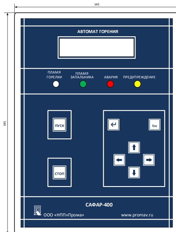
Рис. 8: Панель оператора.
