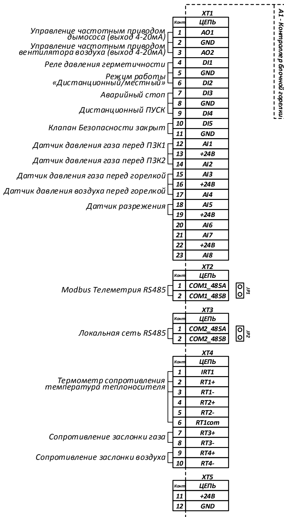
Рис. 1: А1 – Клеммы контроллера автомата.
